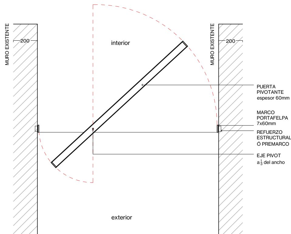
Corte en Planta Superior
