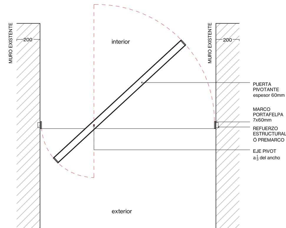
Corte en Planta Superior
